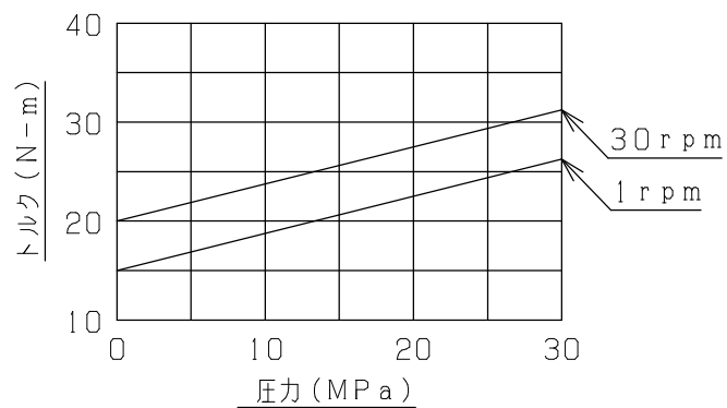
トルク性能表 (実測)
