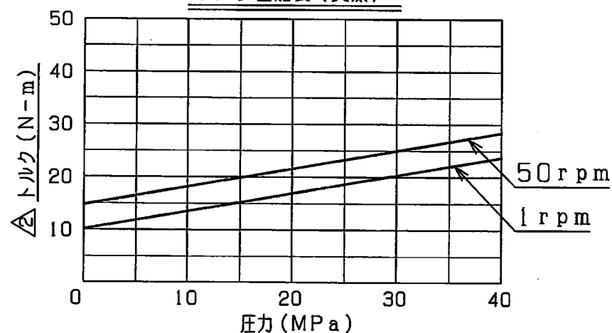
トルク性能表(実測)
