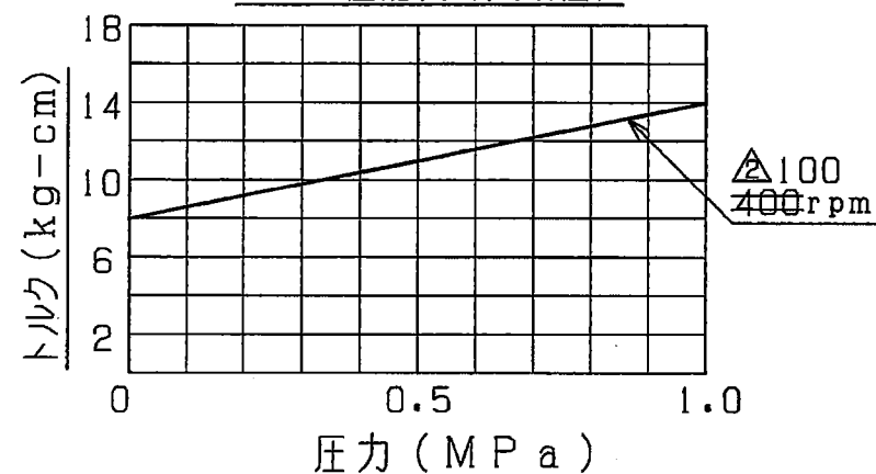
トルク性能表 (実験値)
