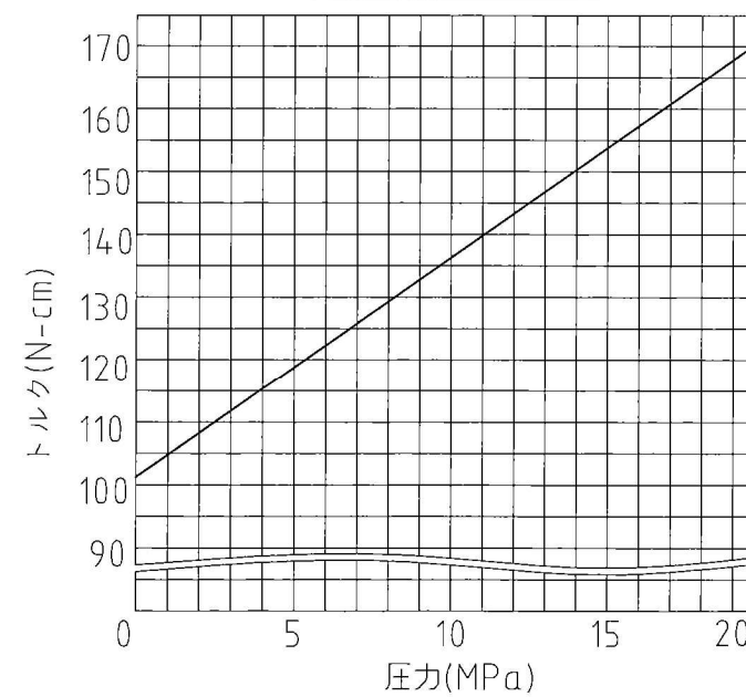
トルク性能表(実測値)
