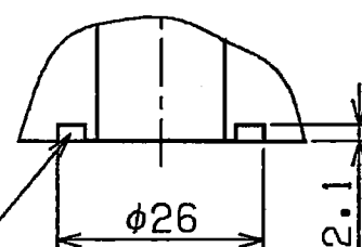
リング溝詳細 (2ヶ所)
