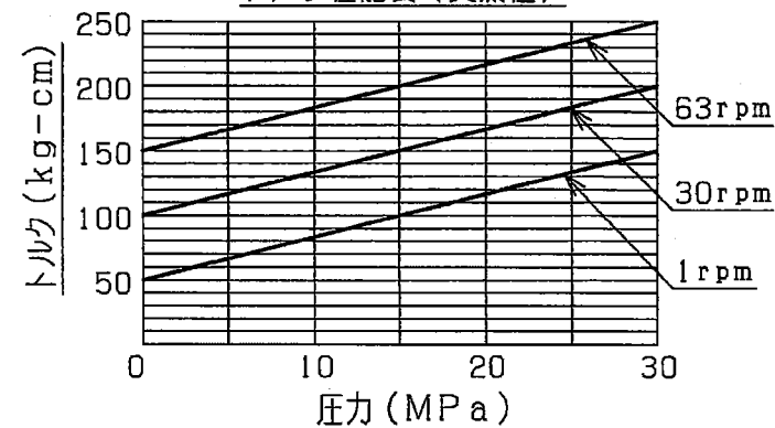
トルク性能表 (実測値)
